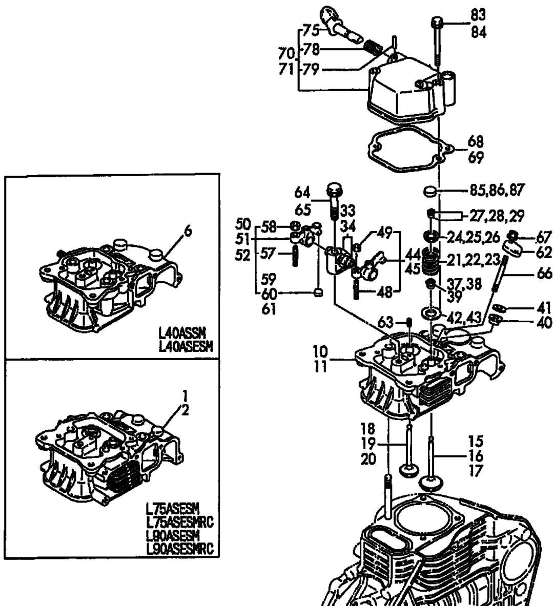
Fig. 2 シリンダヘッド&ボンネット CYLINDER HEAD & BONNET
