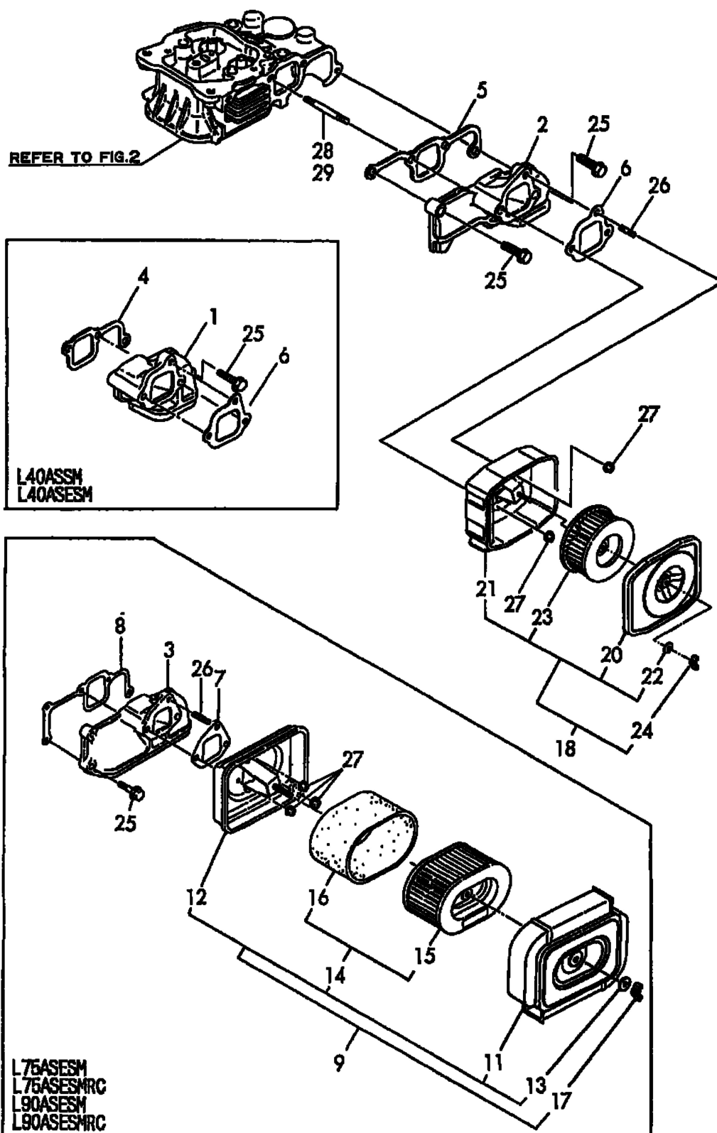
Fig. 3 エアクリーナ AIR CLEANER
