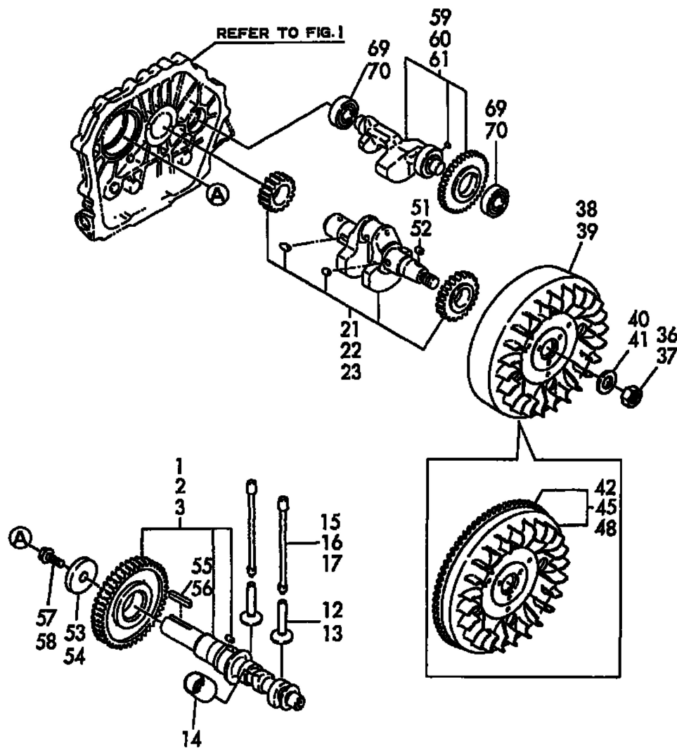
Fig. 5 カムシャフト & クランクシャフト CAMSHAFT & CRANKSHAFT
