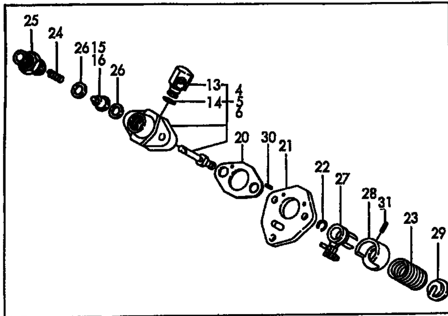
Fig. 9 FOフンシャポンプ FUEL INJECTION PUMP
