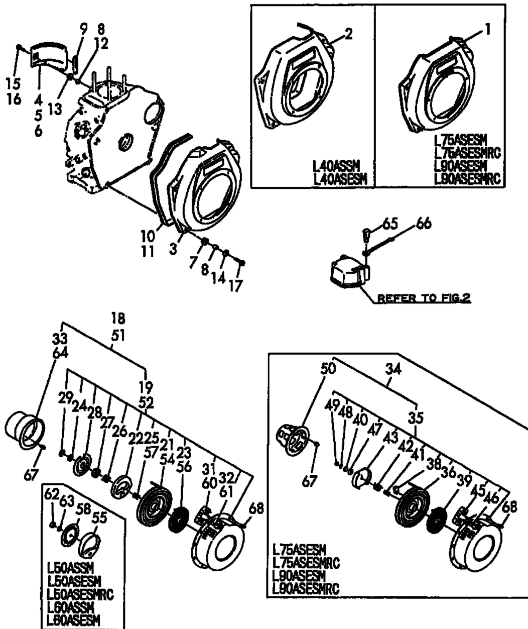
Fig. 8 レイキャク & シドウスウチ COOLING & STARTING DEVICE
