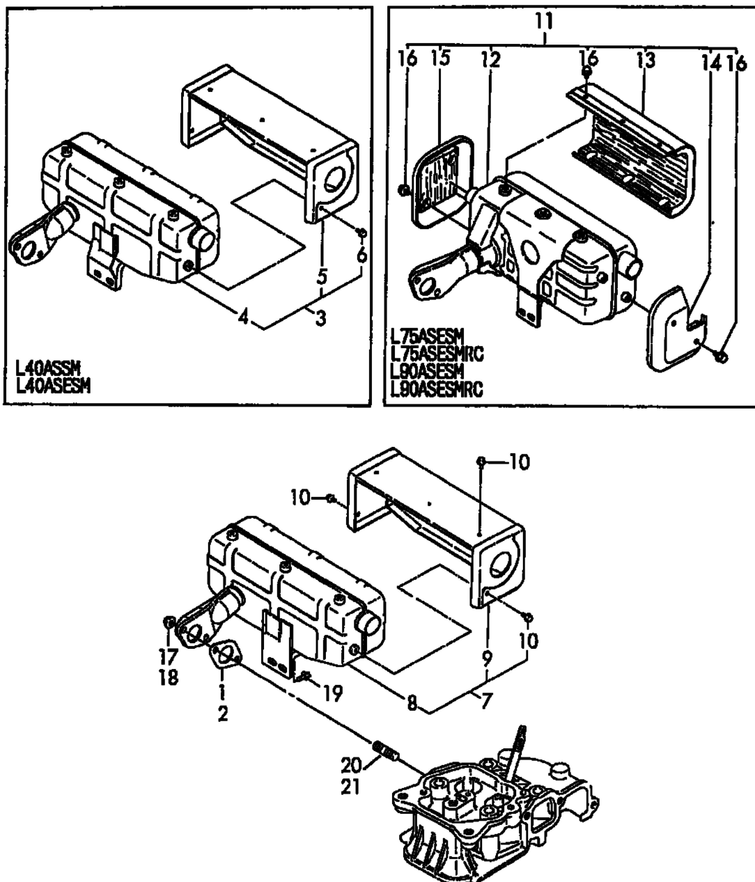
Fig. 4 マフラー MUFFLER
