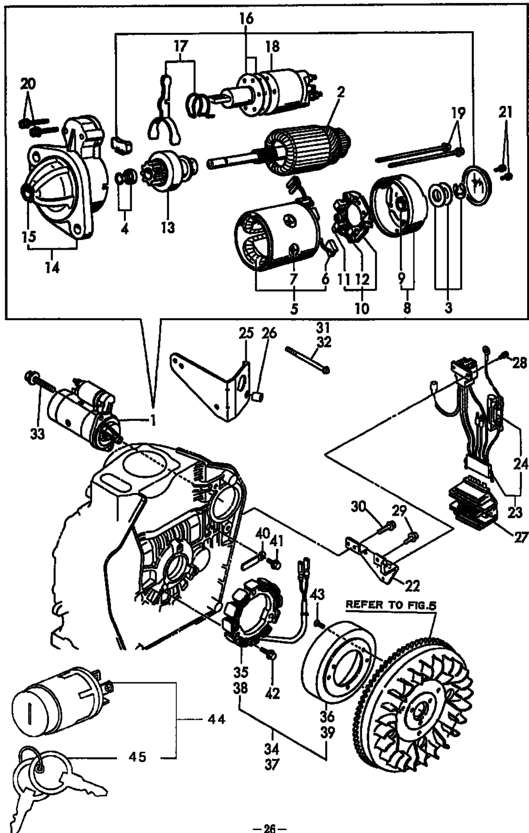
Fig. 11 スタートモーター & ダイナモ STARTING MOTOR & DYNAMO
