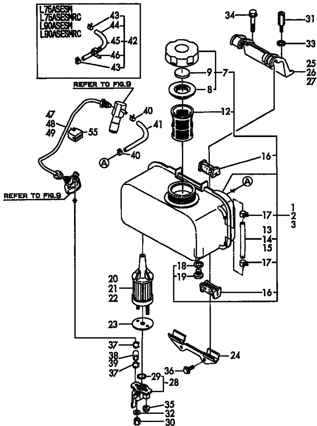
Fig. 10 FOタンク&FOパイプ FUEL TANK & FUEL LINE
