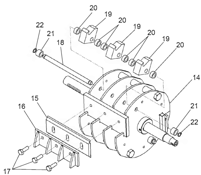
複合ロータ詳細
