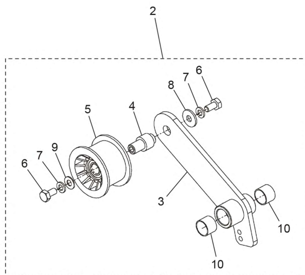
テンションアーム詳細
