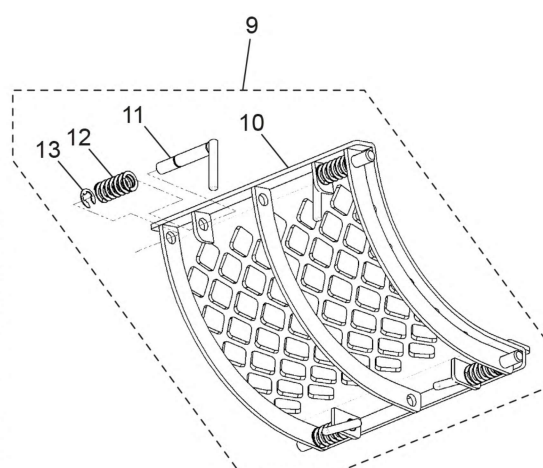
スクリーン詳細
