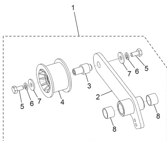
テンションアーム詳細
