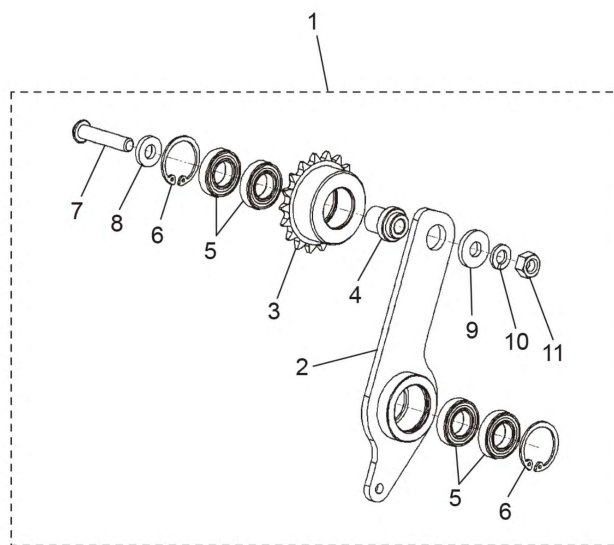
チェーンテンショナ詳細
