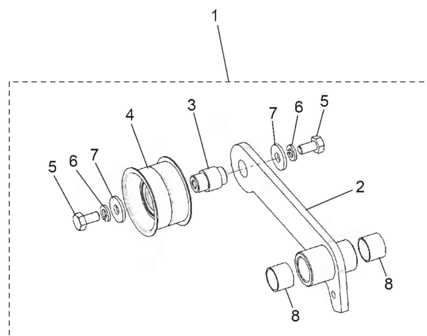
テンションアーム詳細
