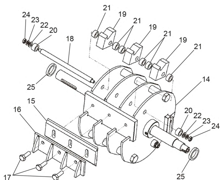
複合ロータ詳細
