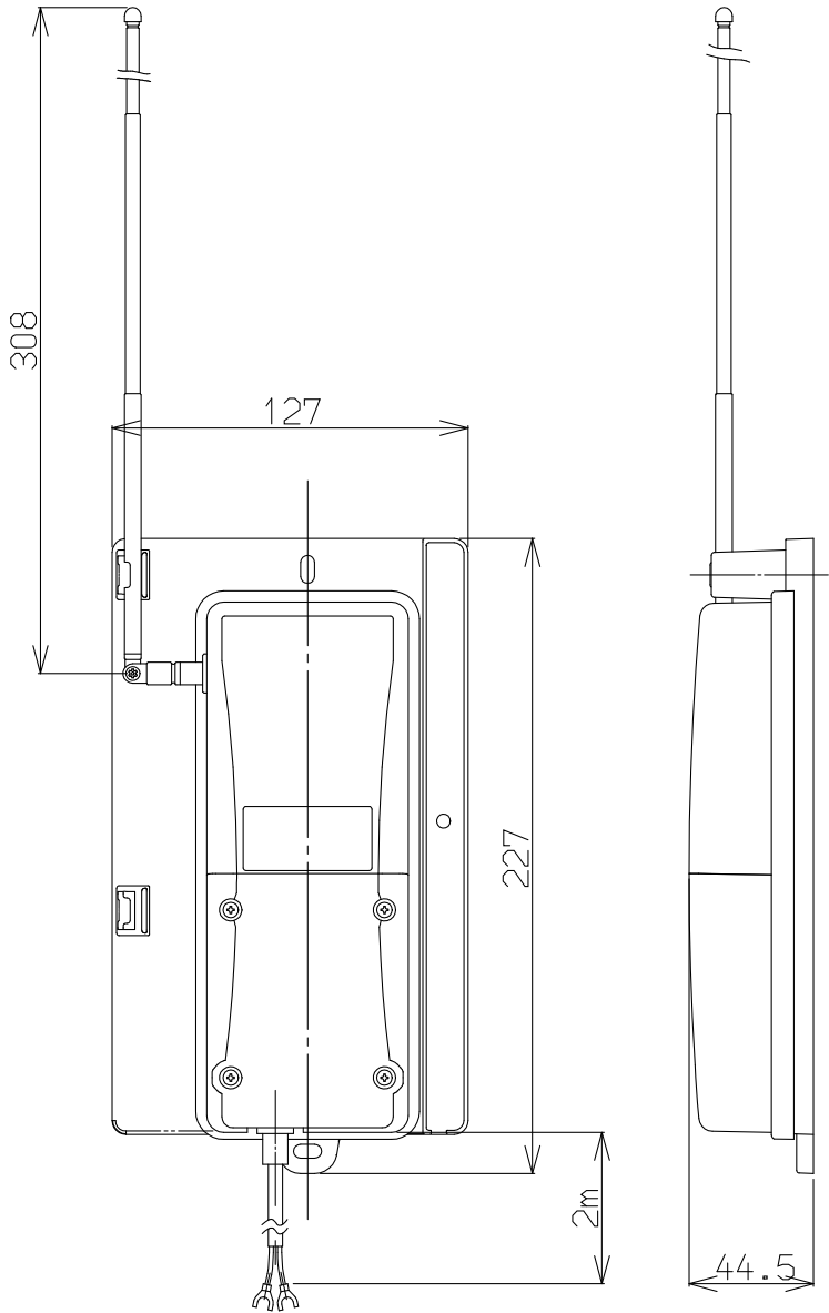
通信ユニット
