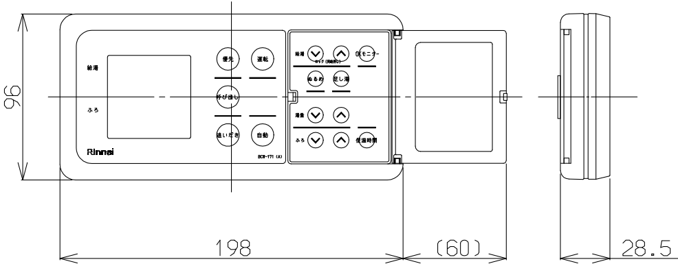
浴室リモコン
