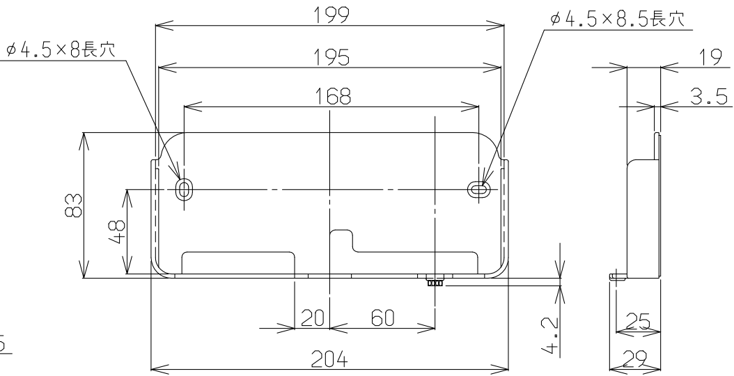
浴室リモコン取付板
