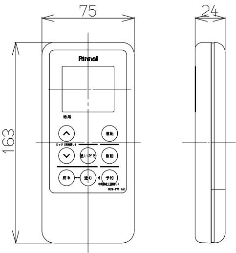
台所リモコン
