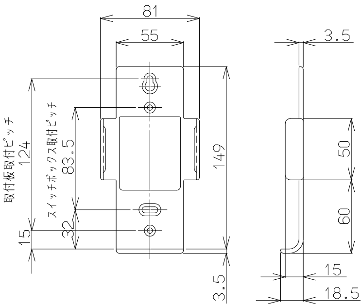
台所リモコン取付板
