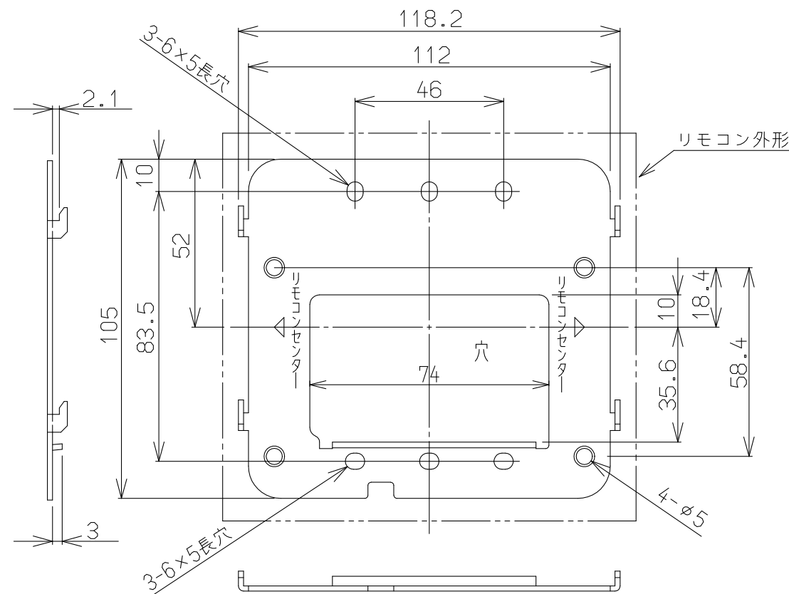
台所リモコンの壁取付金具 (t=1.6)
