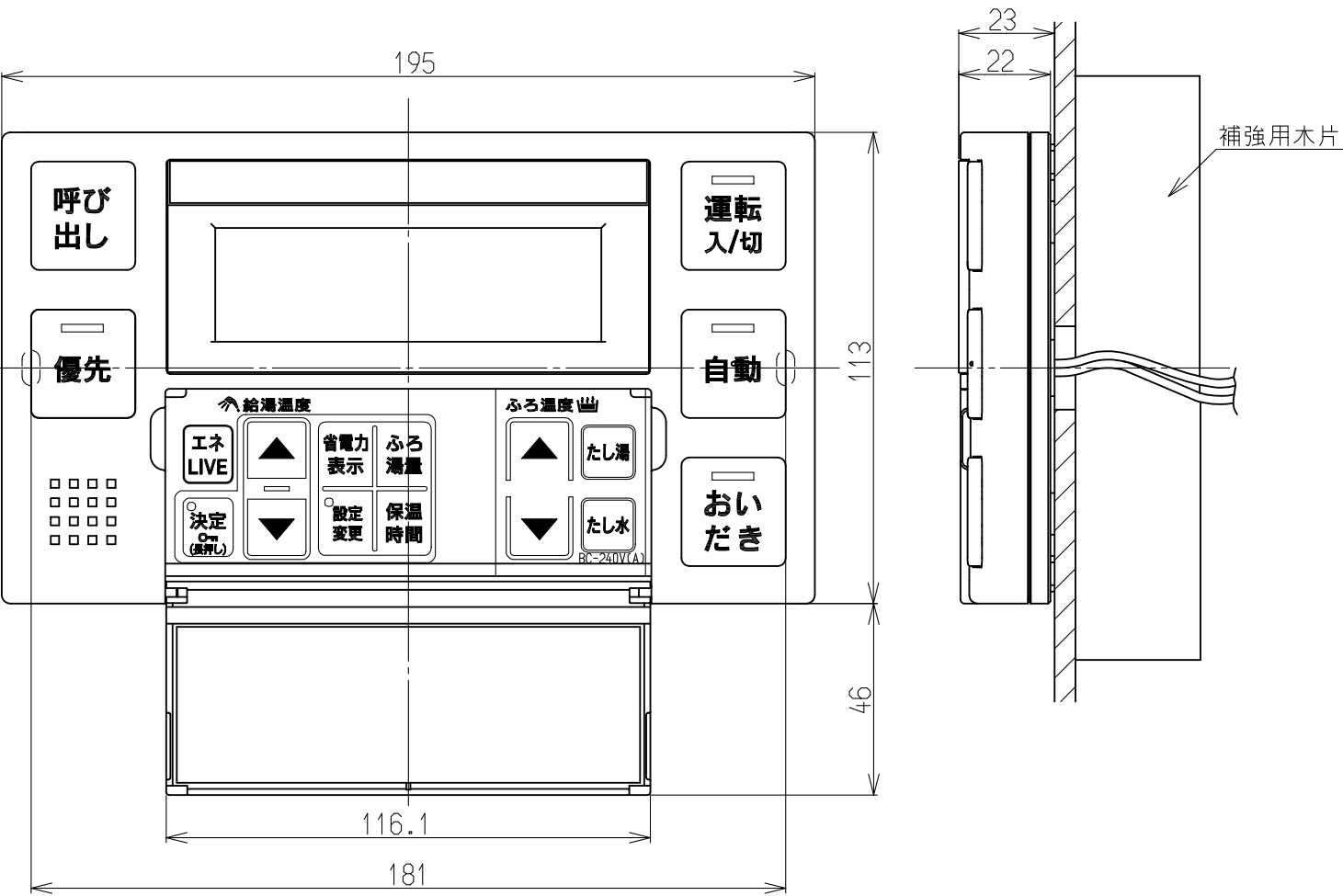
浴室リモコン
