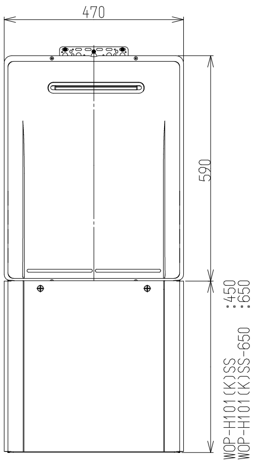
配管カバー取付図(1:10)
