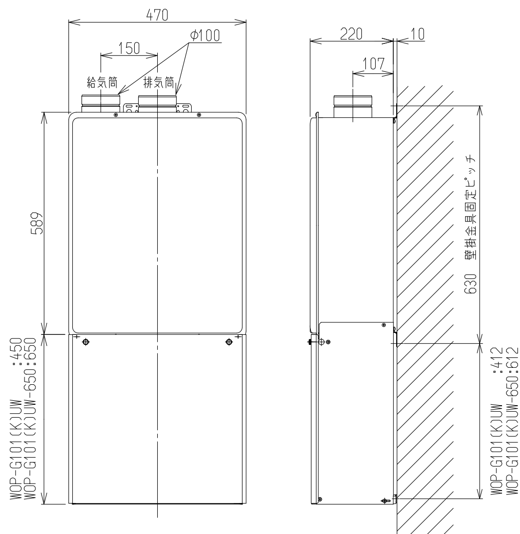
設置図 (S=1:10)
