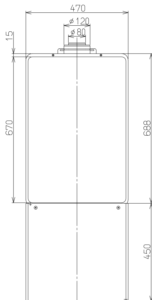
設置図 (S=1:10)
