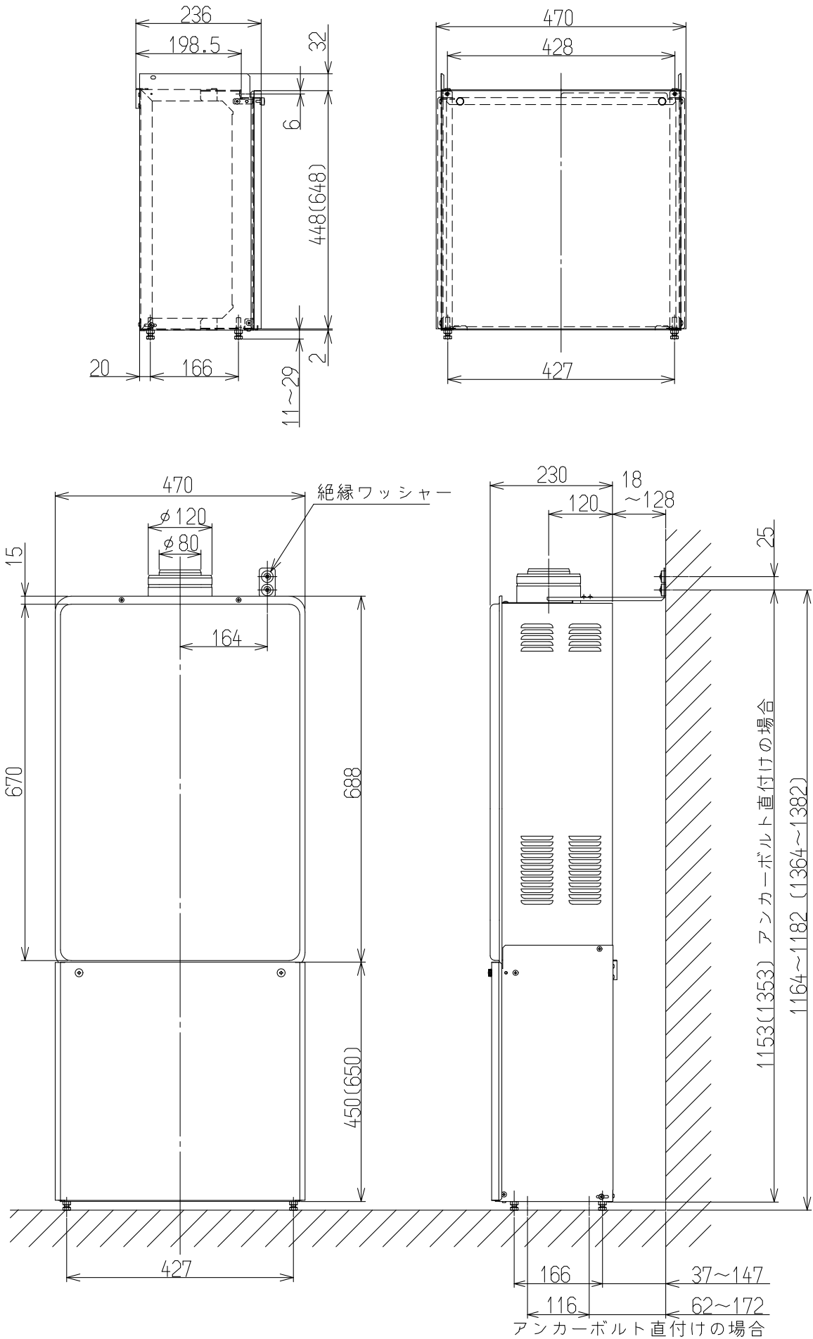
据置台 寸法図
