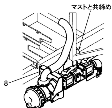
詳細図C
