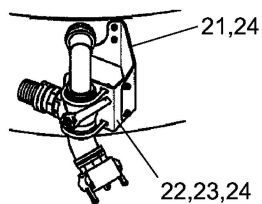
詳細図B
