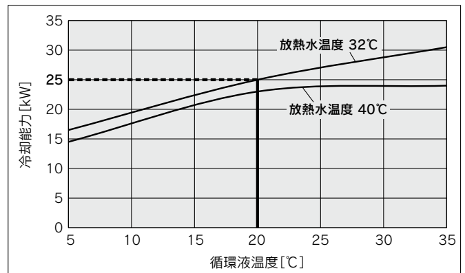
HRSHF250-W□-20/40-□
