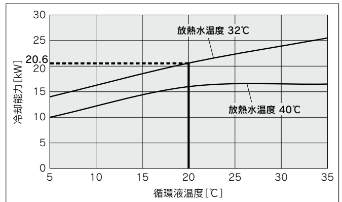
HRSHF250-W□-20/40-□
