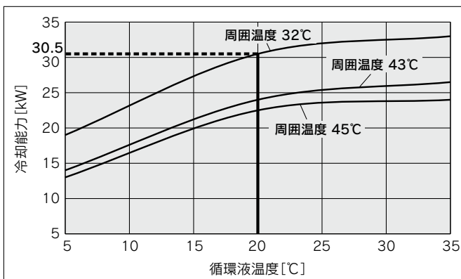
HRSHF300-A□-20/40-□
