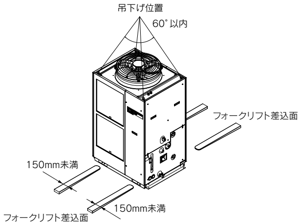
HRSHF250-A-20の場合
