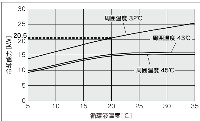
HRSHF250-A□-20/40-□
