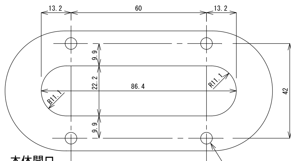
本体開口
