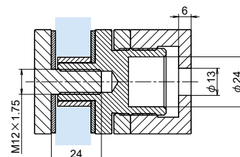
断面図 A-A
