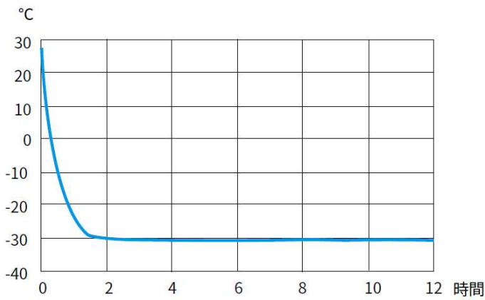
設定温度-30℃までの庫内温度変化
