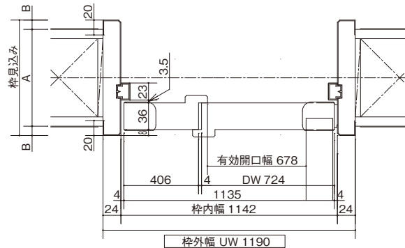
横断面図
