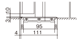
■見切縁納まり111mmタイプ (枠見込み155以上)
