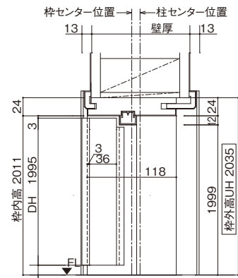
縦断面図
