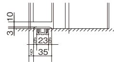
■見切縁納まり35mmタイプ
