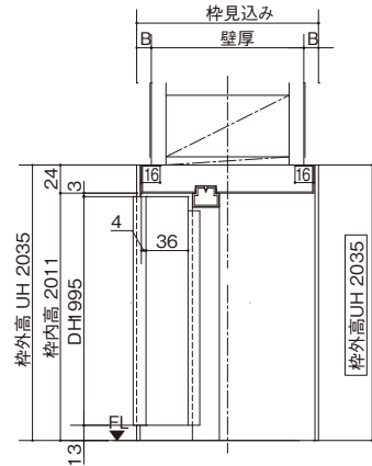
■見切縁納まり111mmタイプ (枠見込み155以上)
