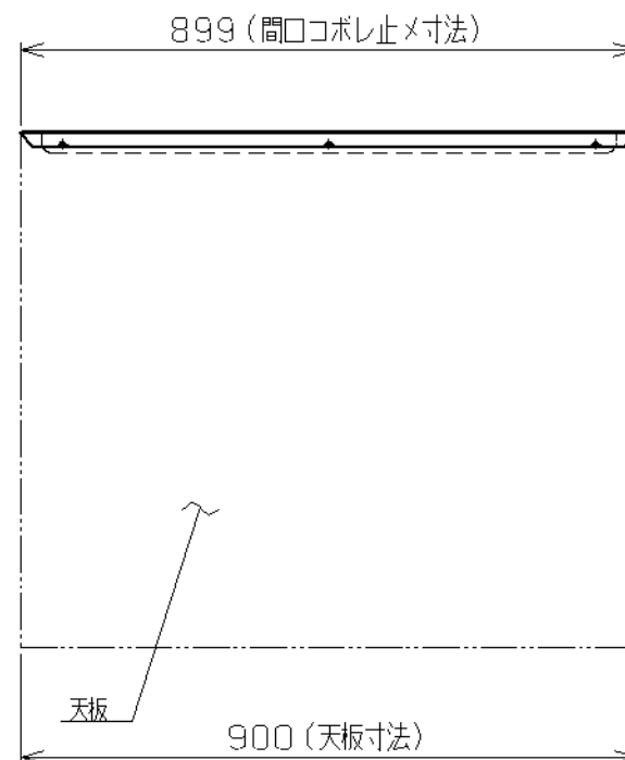
取付例 (S=1/12)
