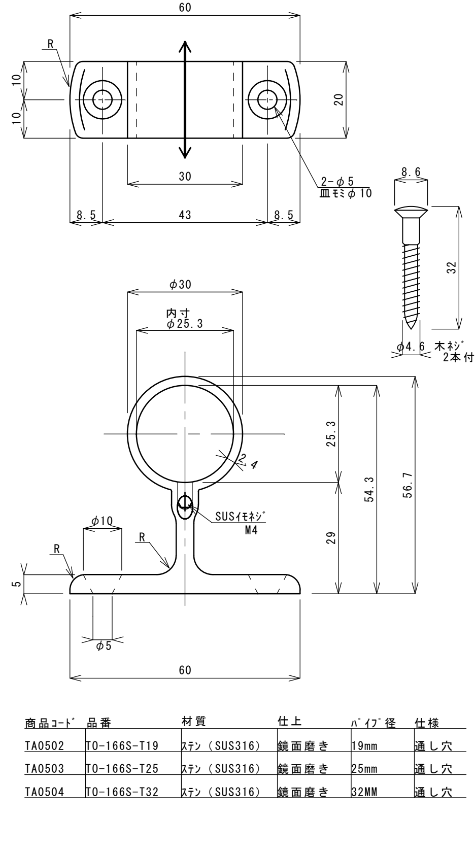
T0-166S-T25
