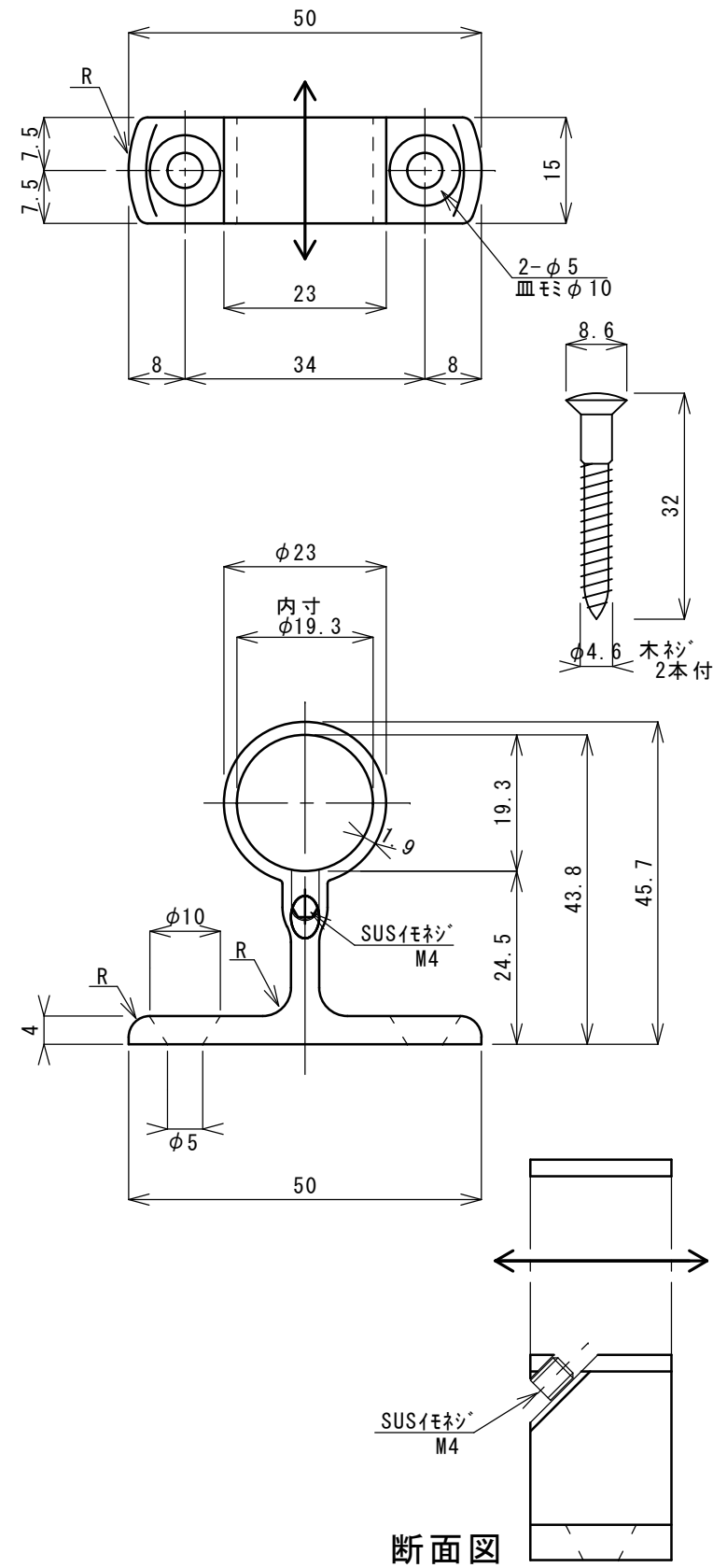
T0-166S-T19
