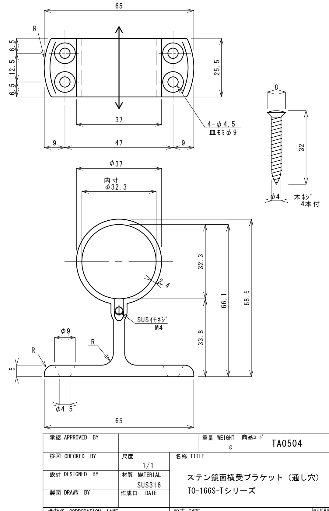
T0-166S-T32
