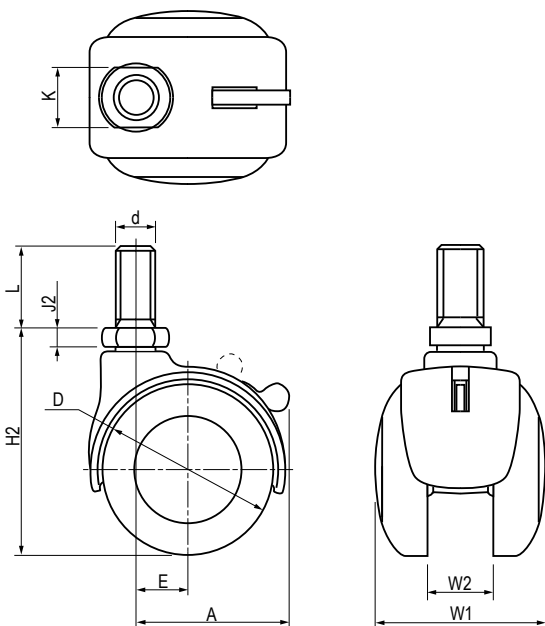
ネジ式 (ストッパー付) Bolt type (with stopper)
