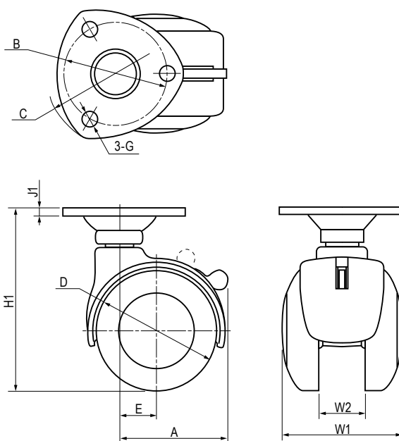
プレート式 (ストッパー付) Plate type (with stopper)
