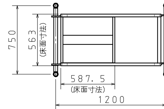
B-B 矢視図 (S=1:25)
