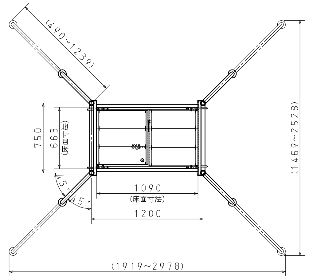
A-A矢視図 (S=1:25)
