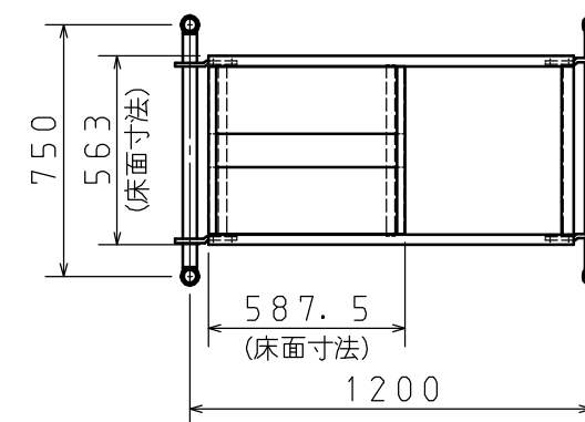
B-B矢視図 (S=1:25)
