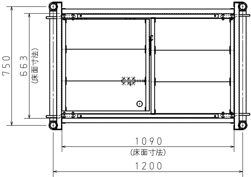
A-A矢視図
