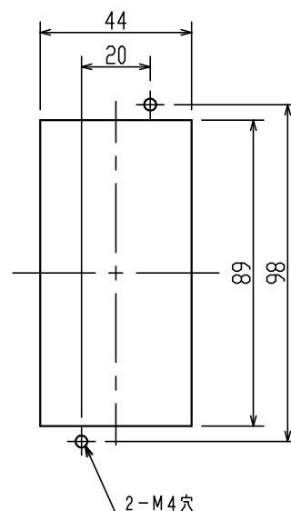
穴明け寸法
