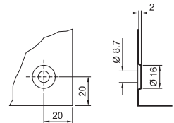
壁面固定部寸法
