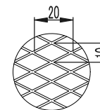
ラス網 10×20 (呼称・3メッシュ)
