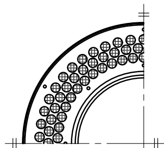
背面図
