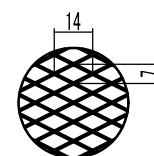
オブション ラシ網 7×14 (呼称・5メッシュ)
