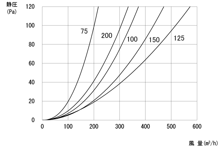
圧力損失曲線
