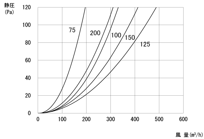
圧力損失曲線
