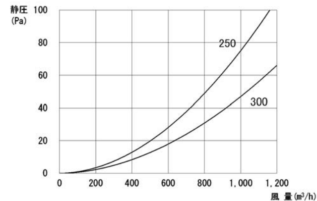
圧力損失曲線
