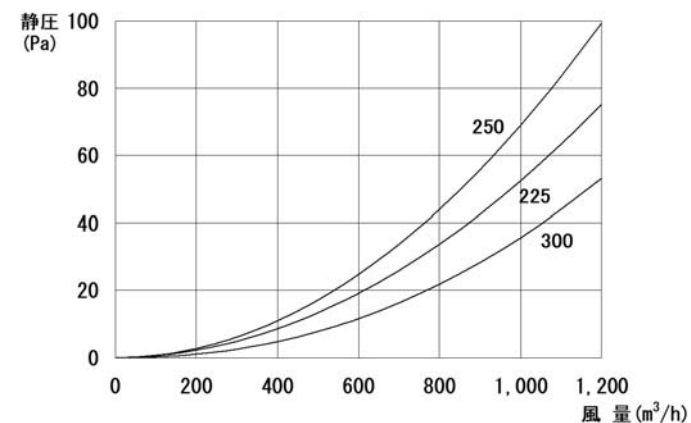
圧力損失曲線
