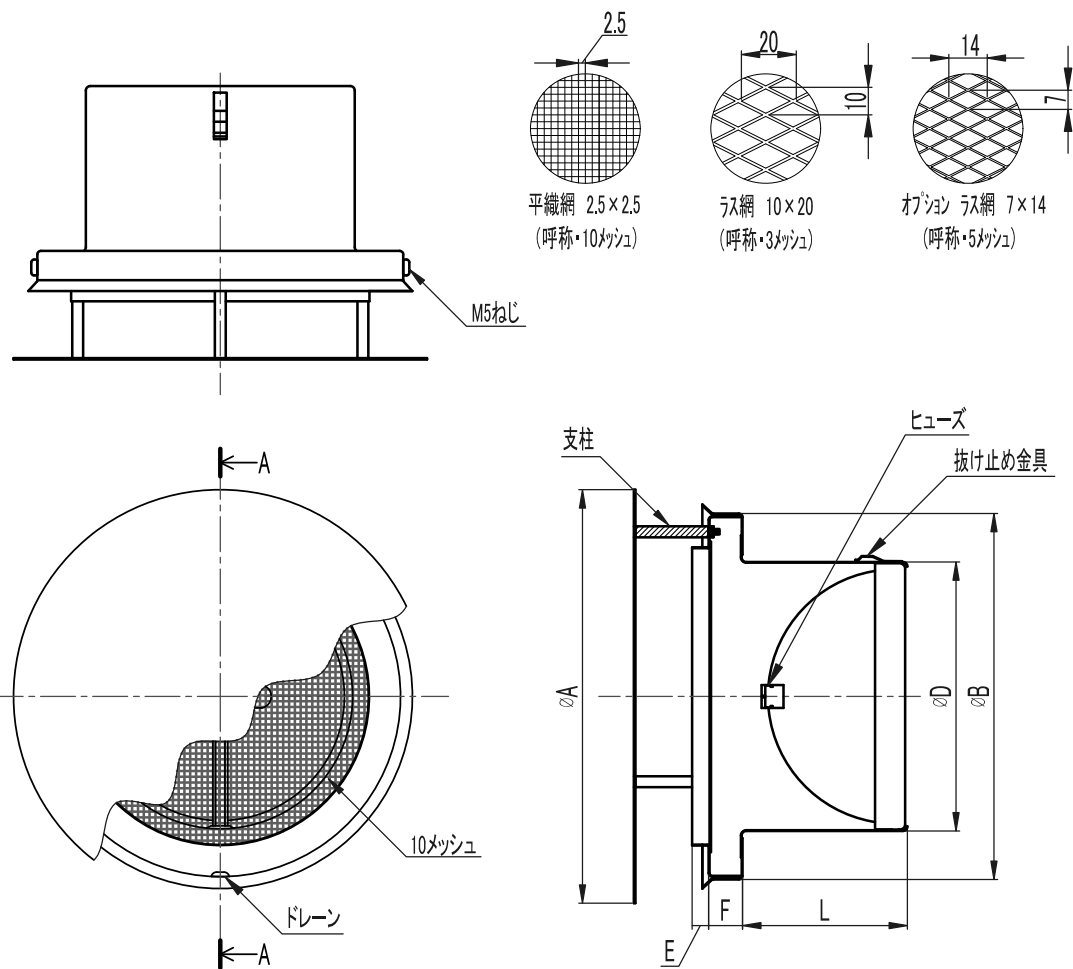
A-A断面図
