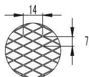
オープンラシ網 7×14 (呼称・5メッシュ)
