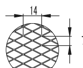
ラシ網 7×14 (呼称・5メッシュ)
