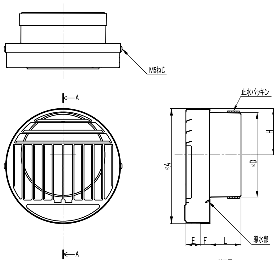
A-A断面図
