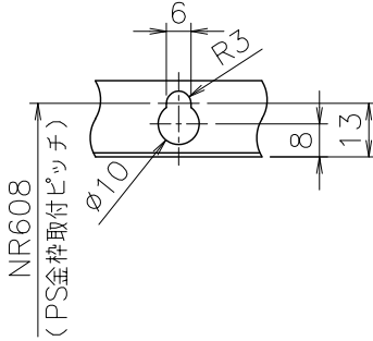
■ウ部詳細図(尺度1/2)
