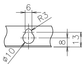
■A部詳細図(尺度1/2)
