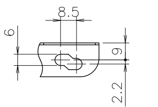
■イ部詳細図(尺度1/2)
