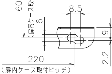
■イ部詳細図(尺度1/2)
