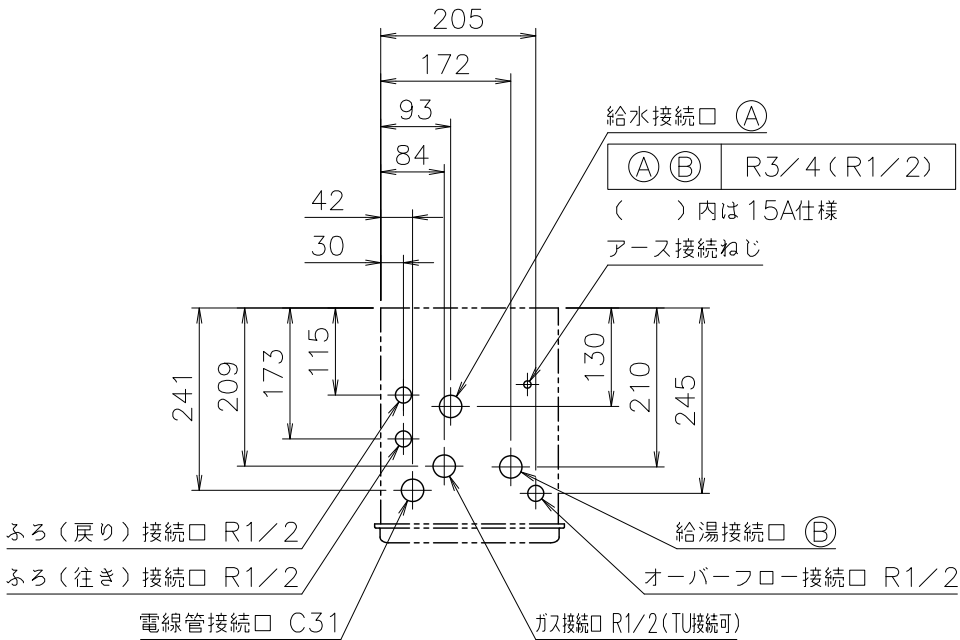
(機器上方よりの透视图)
