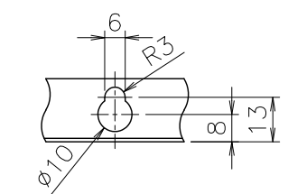
■A部詳細図(尺度1/2)
