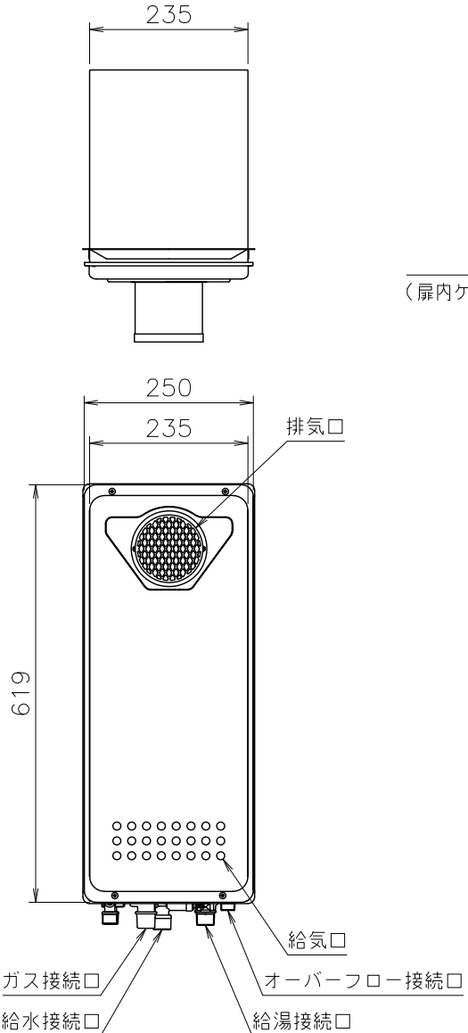
■底板よりの各継手高さ (mm)
